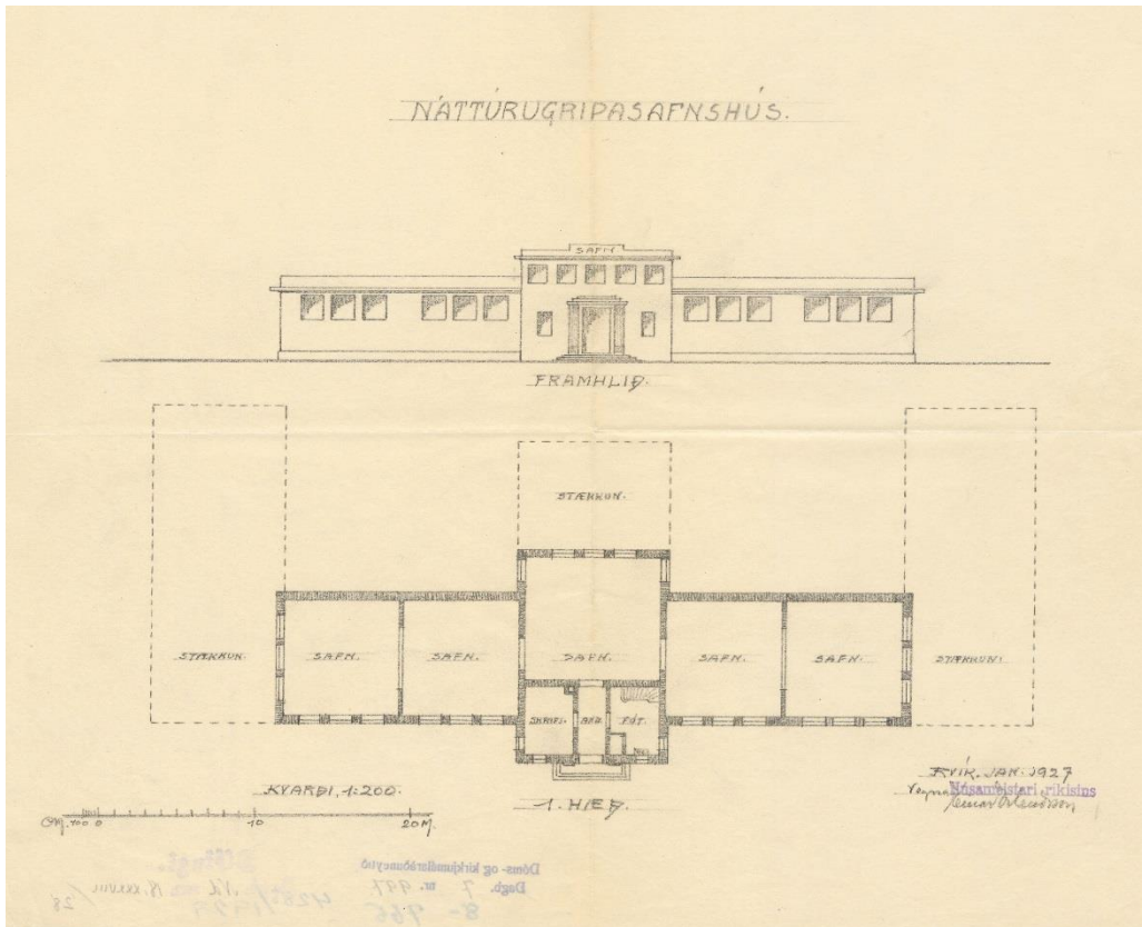
1. mynd. „Náttúrugripasafnshús“, fyrirhugað við hliðina á Safnahúsinu við Hverfisgötu 15, þar sem Þjóðleikhúsið reis síðar. Teikning eftir Einar Erlendsson, aðstoðarmann Guðjóns Samúelssonar húsameistara ríkisins. Dagsett í janúar 1927.
